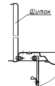
Рисунок 7 – Крепление щитка
