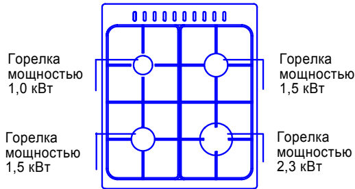
Рис. 12. Верхняя панель плит ЭГ401-2у, ЭГ 401 СТ-2у
