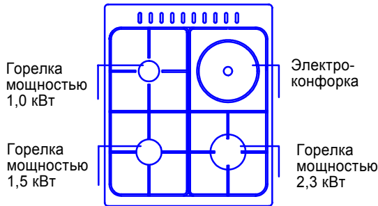
Рис. 13. Верхняя панель плит ЭГ1/3г01-2у
