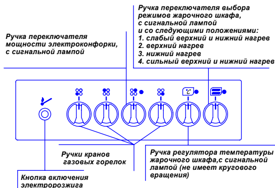
Рис. 11. Передняя панель плиты ЭГ1/3г01-2у
